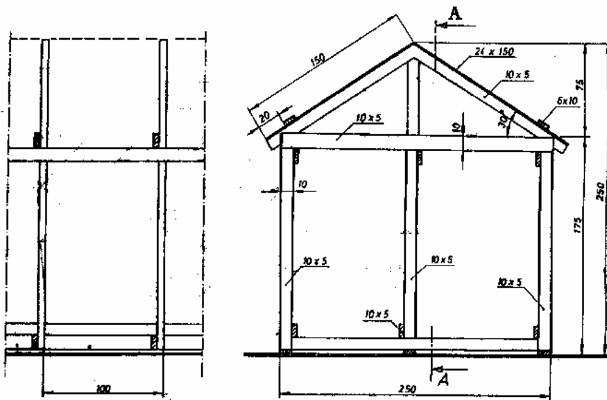
ДЕТАЛЬ А-А
